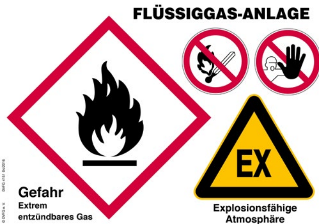
Abb. 16 Sicherheitskennzeichen Flüssiggasanlagen bei Versorgung aus ortsfesten Druckgasbehältern (Quelle: DVFG)
