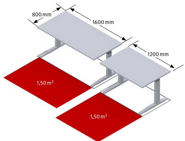
Abb. 8 Bewegungsflächen an Arbeitstischen
