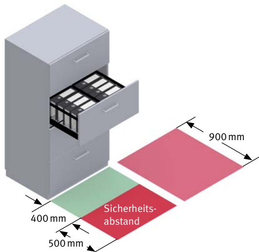
Abb. 12 Ermittlung der Benutzerfläche an einem Schrank mit Auszügen
