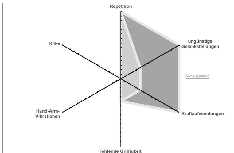
Abb. 42 Spinnendiagramm Statorfertigung
