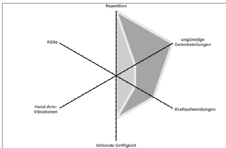
Abb. 37 Einlegeplatz Schweißstrecke
